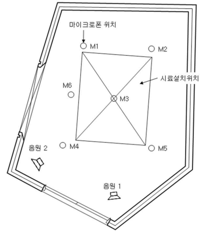
[그림 1] 잔향실 배치도
