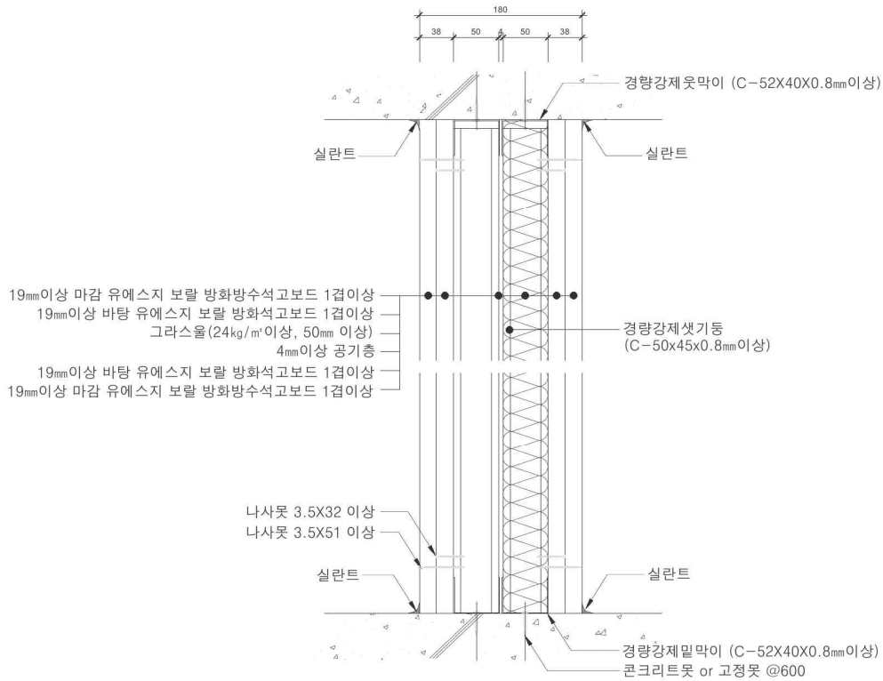
<수직단면도>
