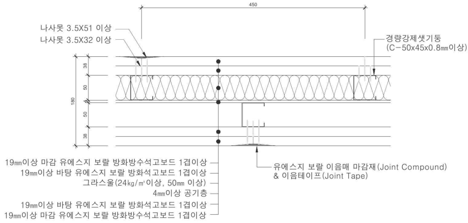
<수평단면도>
