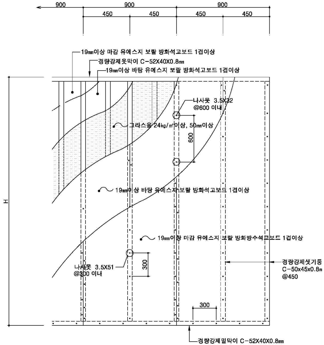
<입면도>
