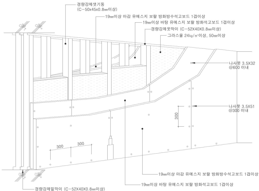
<투시도>
