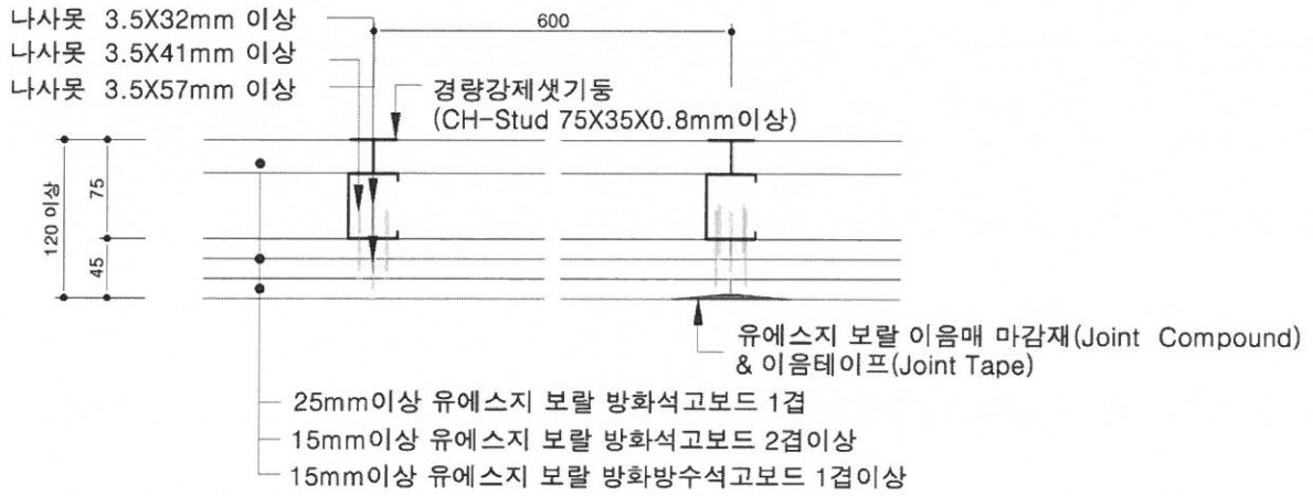
[수평단면 상세도]
