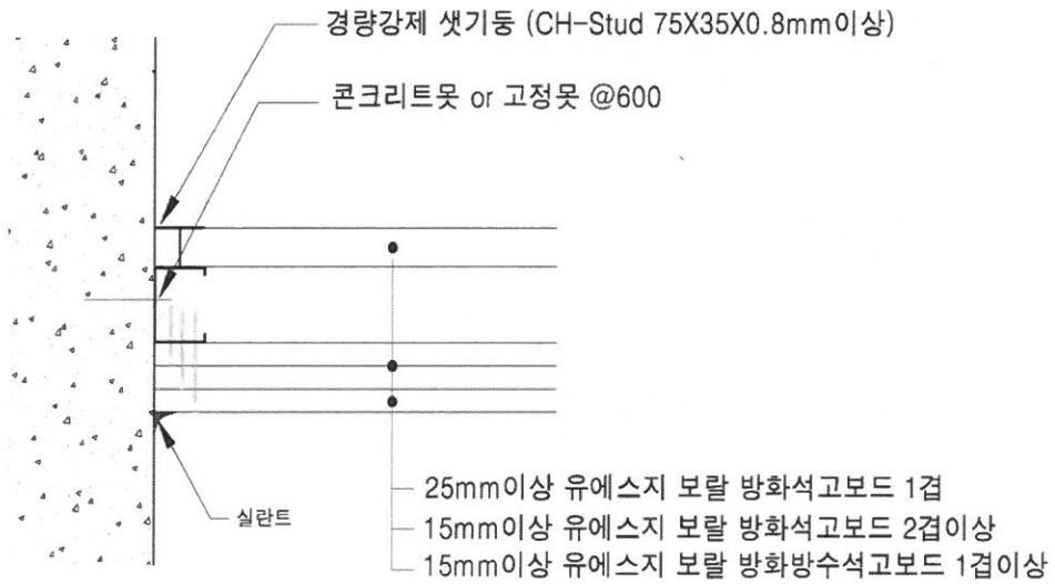
[ 벽 접합 상세도 ]
