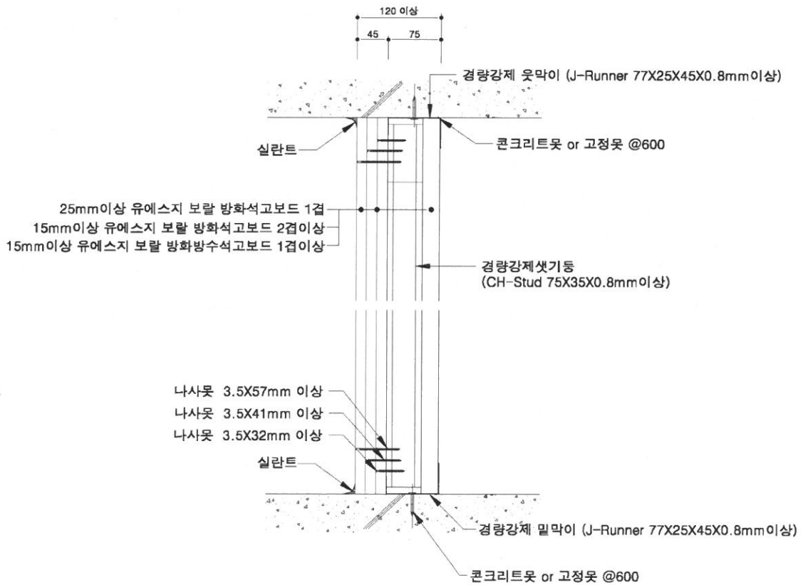
[수직단면 상세도]
