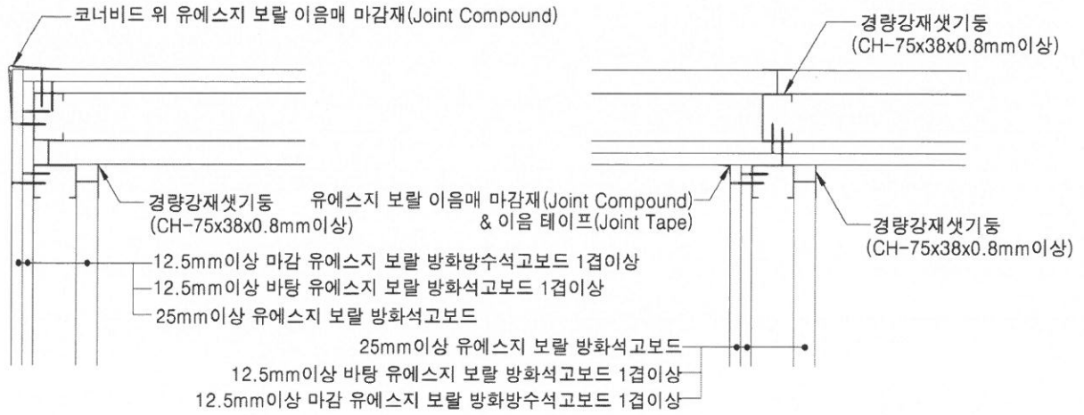
[ “ㄱ” / “T” 접합부위 상세도 ]
