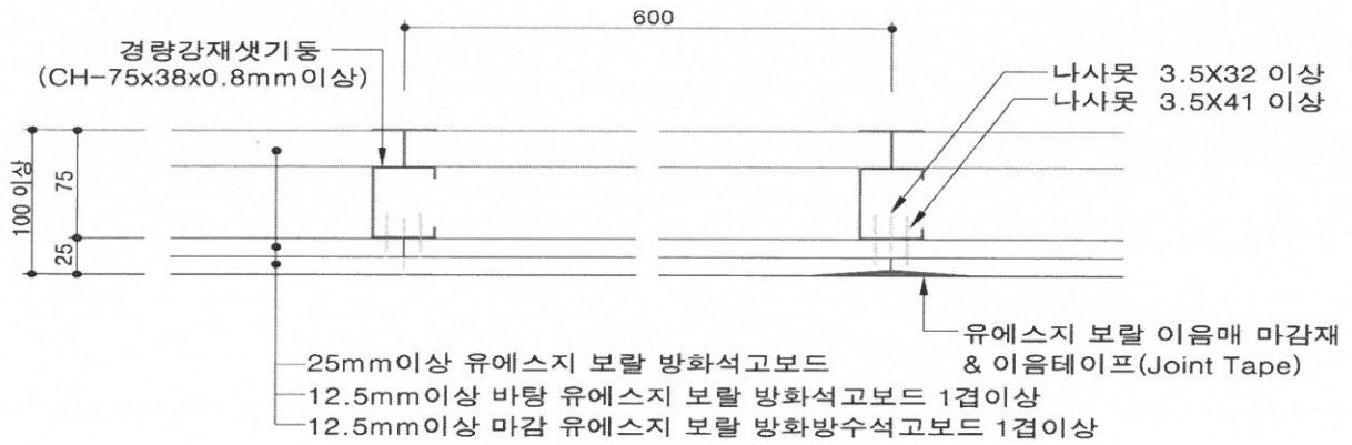
[수평단면 상세도]
