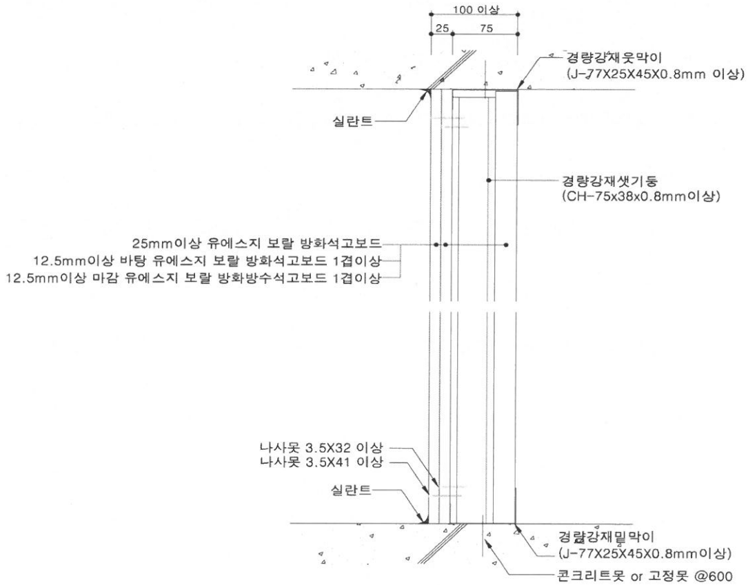
[수직단면 상세도]
