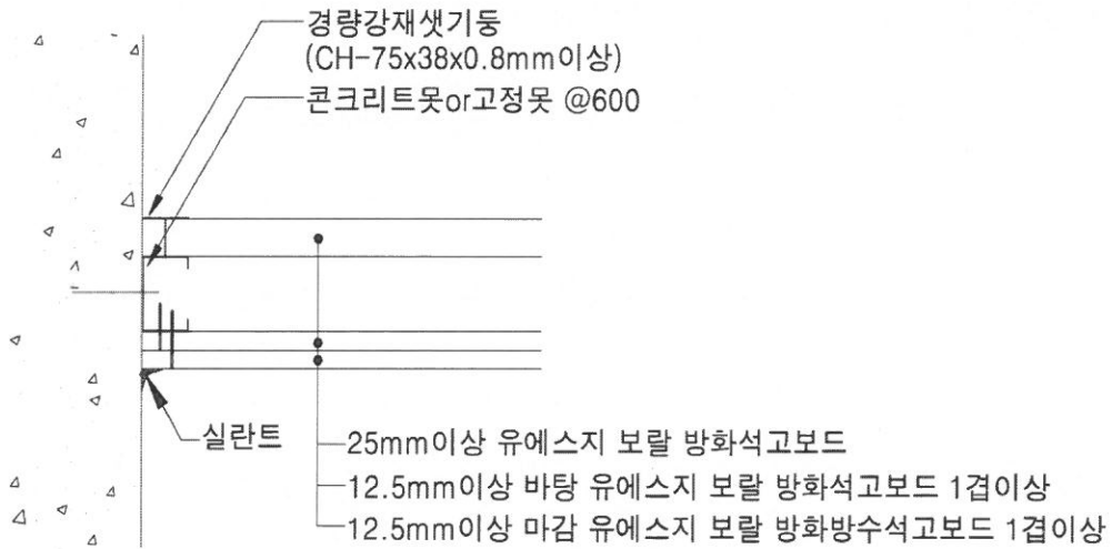
[ 벽 접합 상세도 ]
