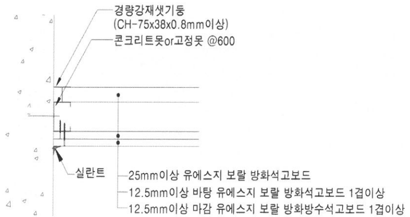
다. 벽 접합 상세도
