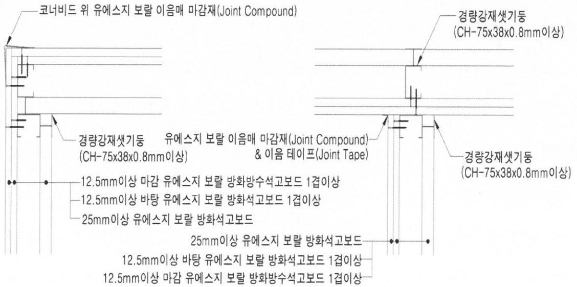
가. “L”접합상세도
