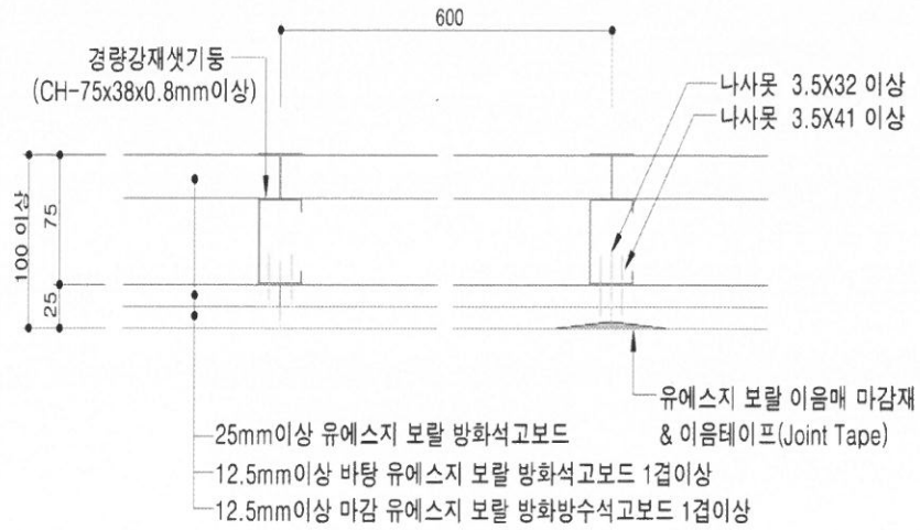
가. 수평 단면도
