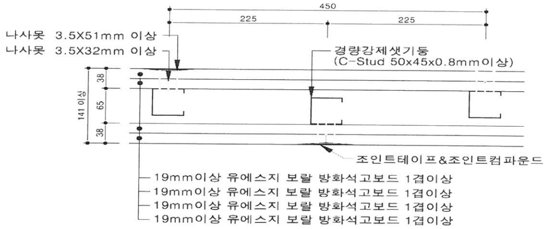
[수평단면 상세도]
