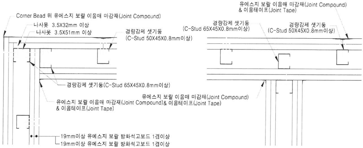
[ “ㄱ” / “T” 접합부위 상세도 ]
