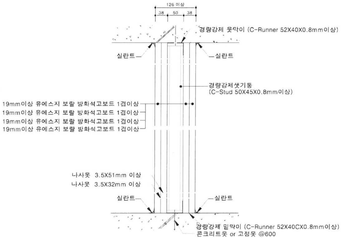
[수직단면 상세도]
