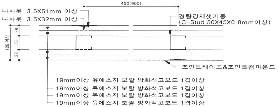
[수평단면 상세도]
