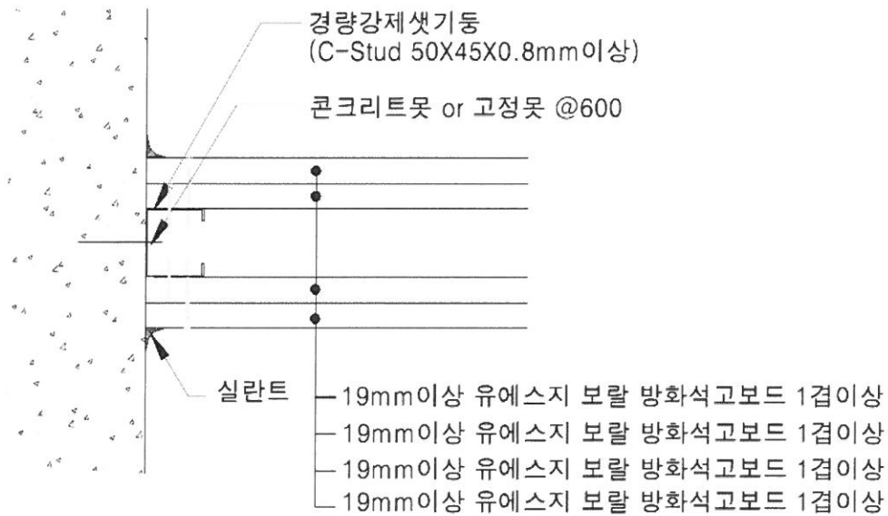
[ 벽 접합 상세도 ]
