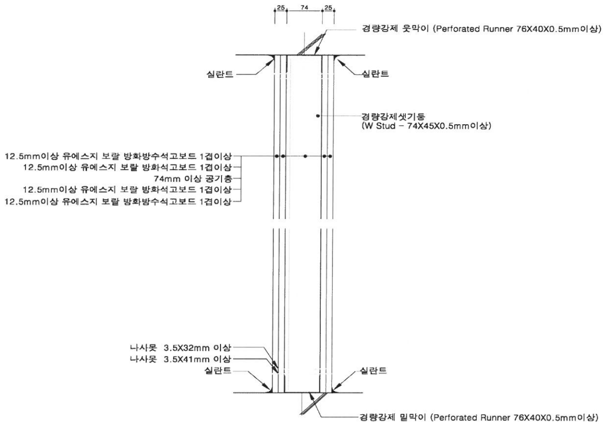
[수직단면 상세도]
