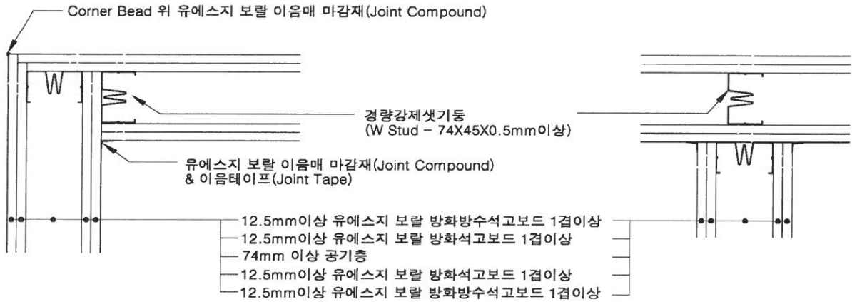
[ “┌” / “T” 접합부위 상세도 ]
