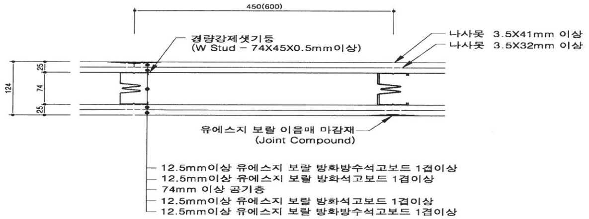
[수평단면 상세도]
