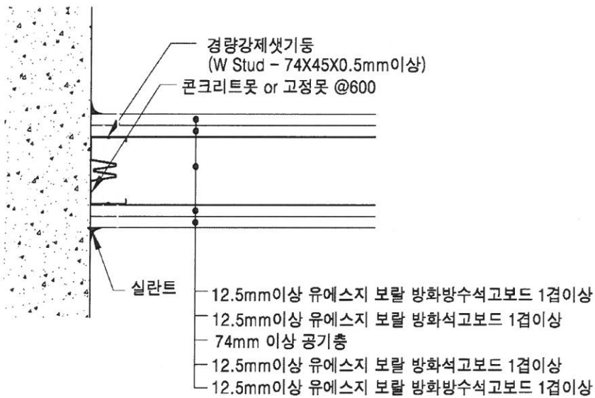
[ 벽 접합 상세도 ]
