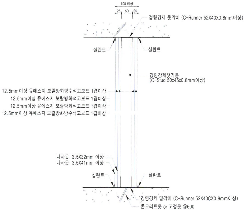
[수직단면 상세도]
