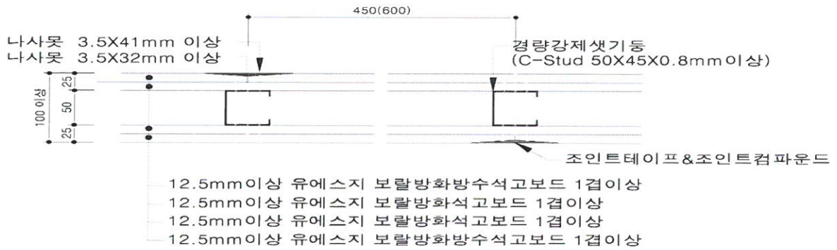
[수평단면 상세도]
