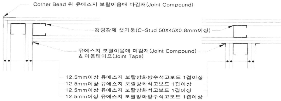
[ “ㄱ” / “T” 접합부위 상세도 ]
