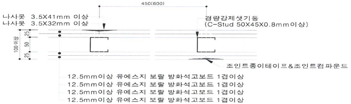
[수평단면 상세도]
