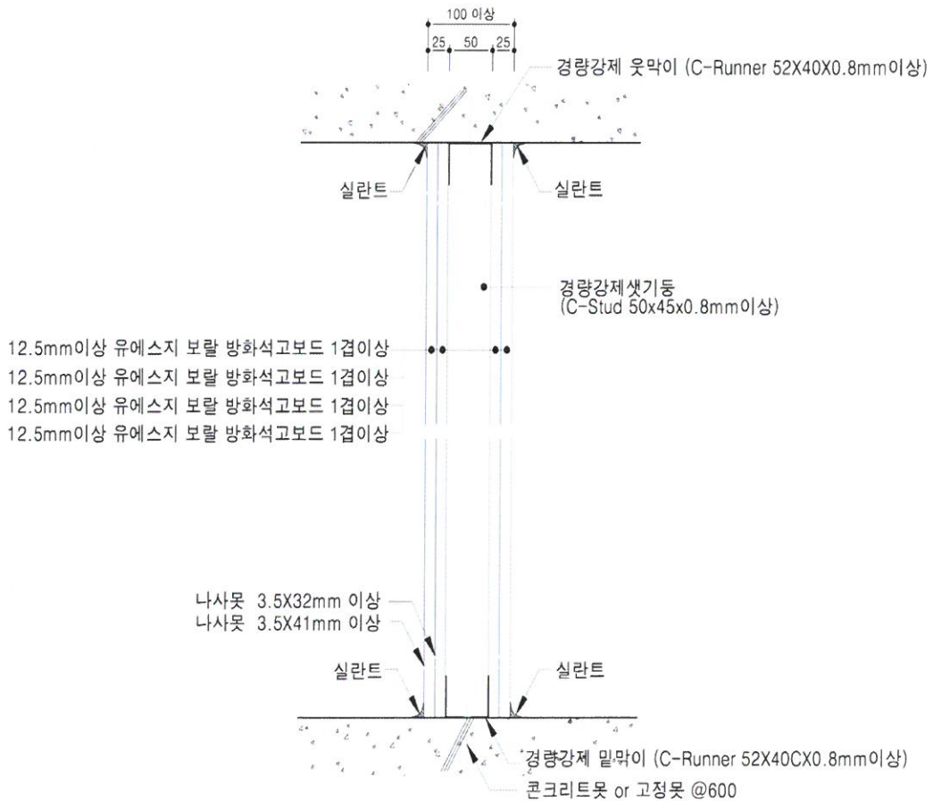
[수직단면 상세도]
